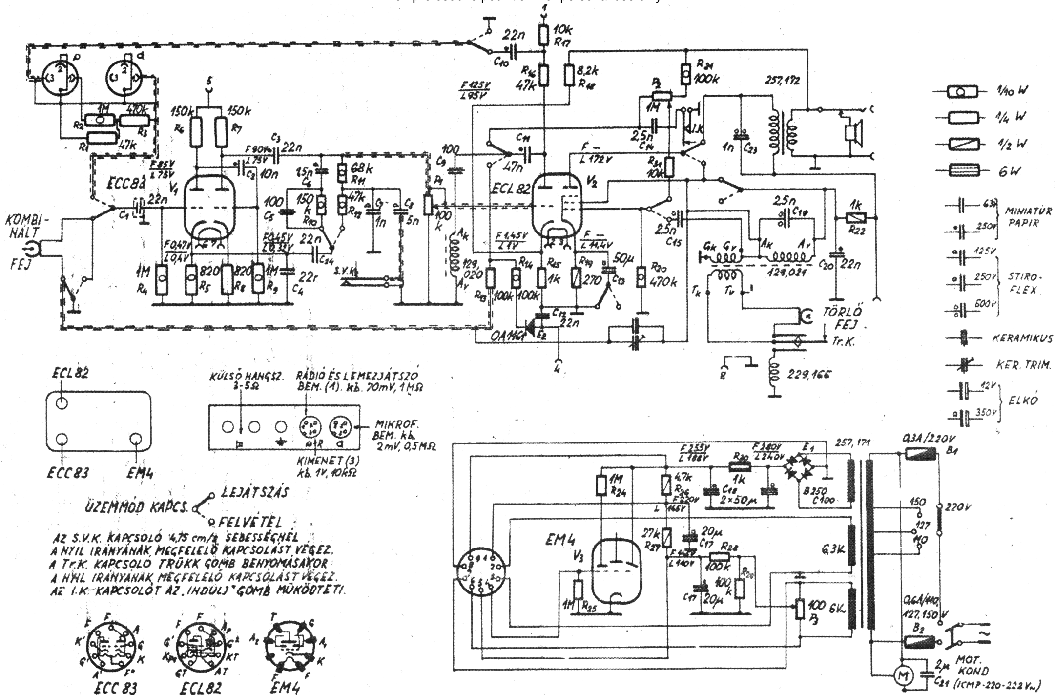
3. ábra. A „TERTA-922” típusú magnetofon kapcsolási rajza
