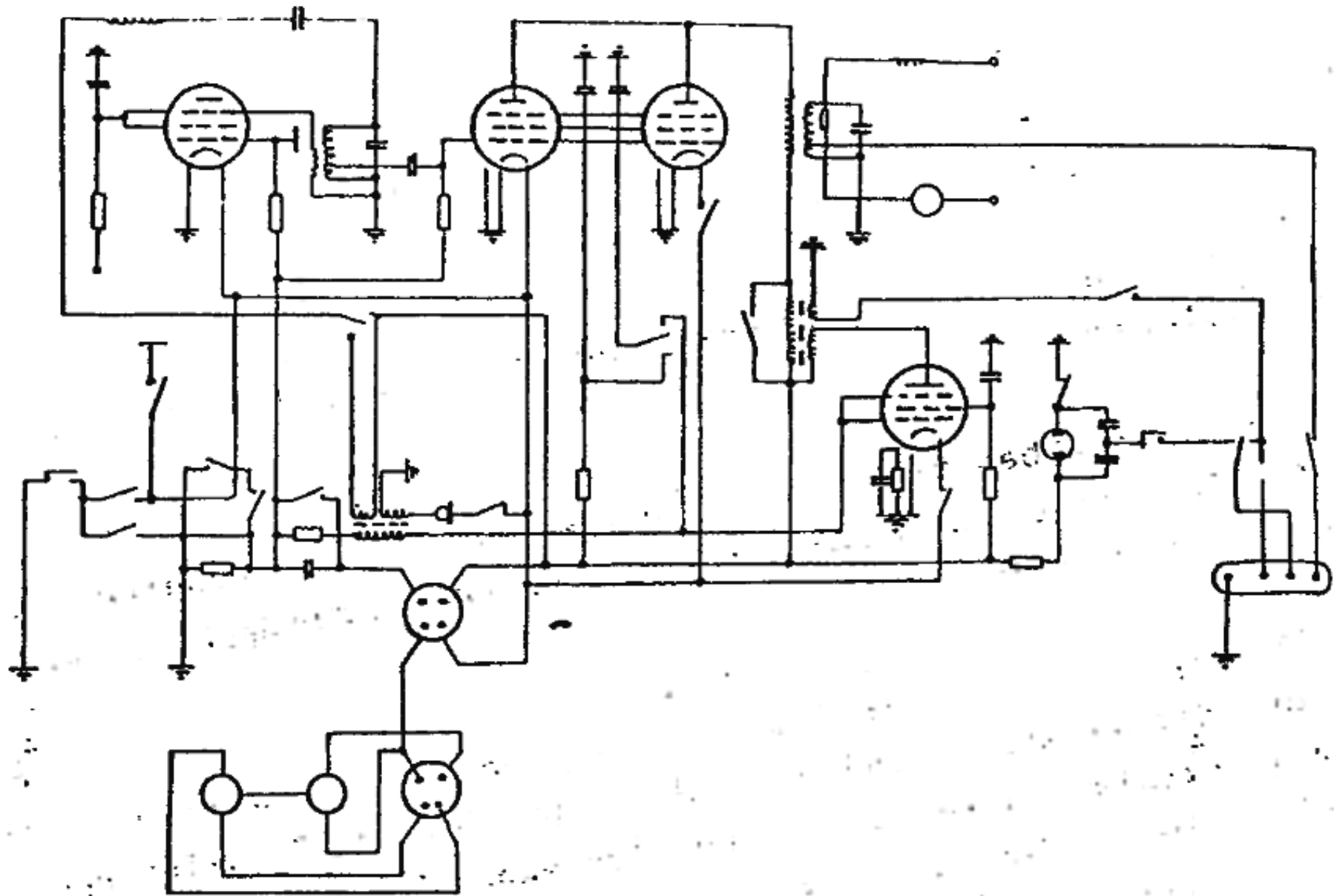
3. ábra. Az R/7a adó kapcsolási rajza
